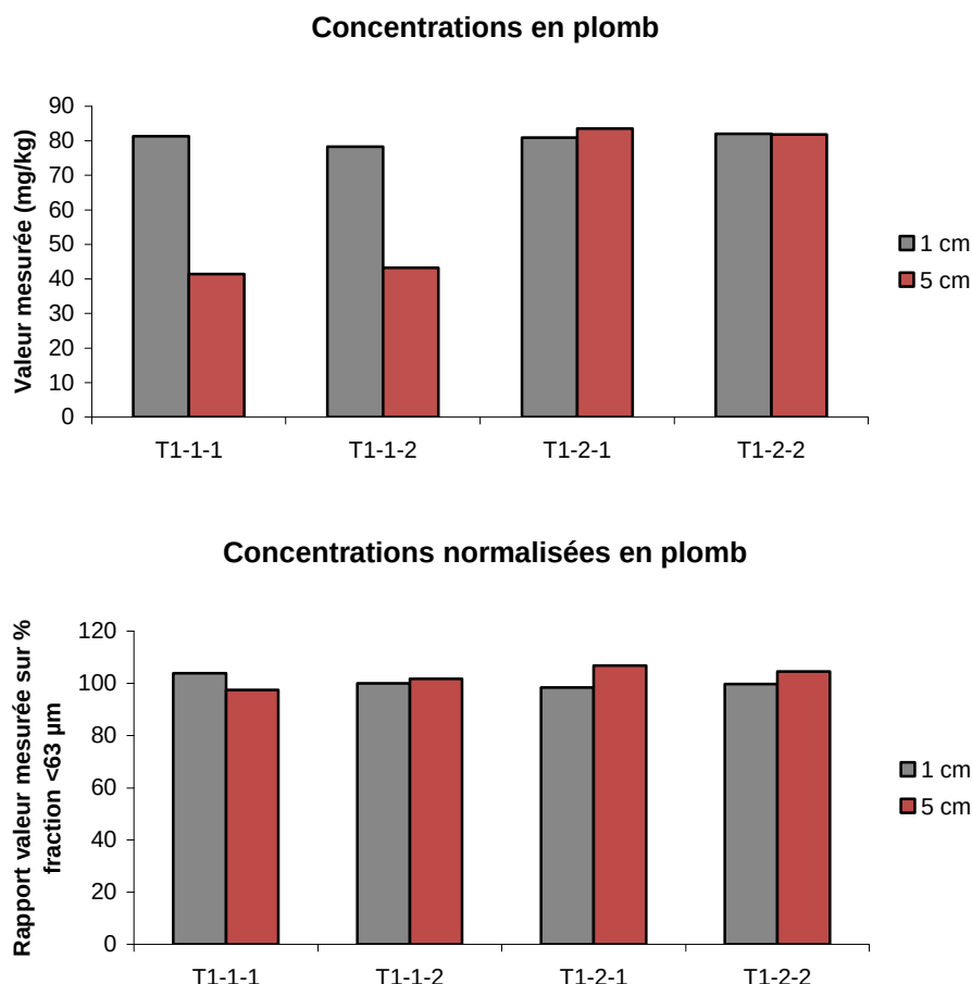
Figure 3 : Comparaison entre les concentrations en plomb mesurées au transect 1 sur le sédiment d'épaisseur 1 cm et 5 cm et ces mêmes concentrations normalisées par la granulométrie
