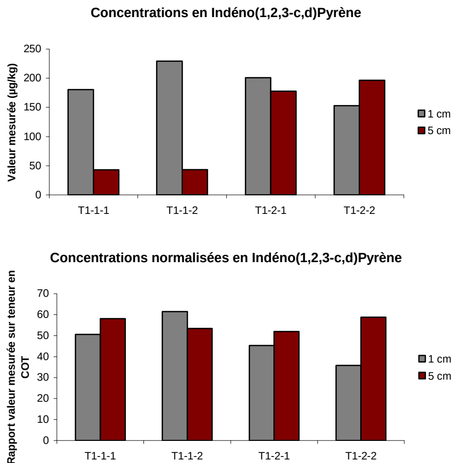
Figure 5 : Comparaison entre les concentrations en indéno(1,2,3-c,d)pyrène mesurées au transect 1 sur le sédiment d'épaisseur 1 cm et 5 cm, et ces mêmes concentrations normalisées par le COT
