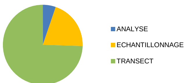
Figure 4 : Représentation de la part de la variance totale due à l'« analyse », à l'« échantillonnage » et au « transect » pour le plomb, sans normalisation des concentrations (cas pour 4 transects - T1 à T4 - et cas pour 3 transects - T2 à T4) et après normalisation des concentrations (4 transects).
