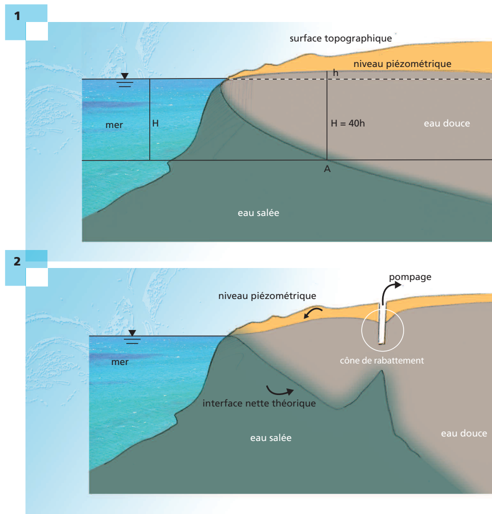
Figure 1. Coupe schématisique perpendiculaire au littoral montrant l'intrusion saline selon Ghyben-Herzberg (extrait de Frissant 2005). Le biseau d'eau salée rentre à l'intérieur des terres et atteint une profondeur H sous le niveau de la mer au point A où la cote piézométrique h est telle que H = 40h .
